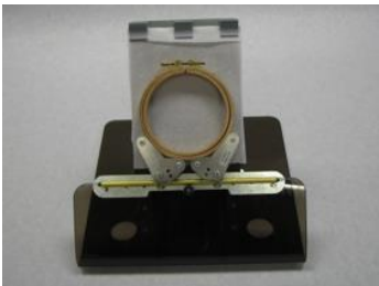
Ärmel/Hosen Einspannvorrichtung
