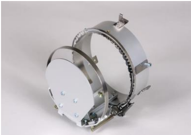
Kappenstick-Einrichtung
