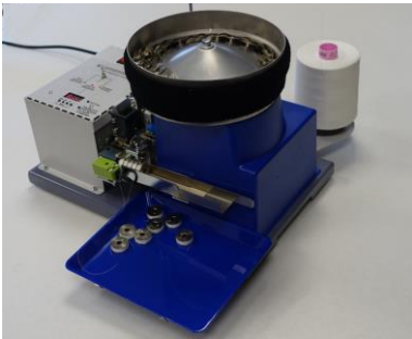
Unterfaden-Spulautomat
