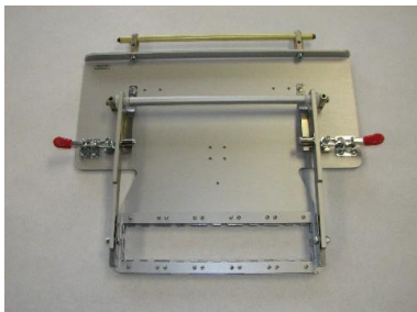
Pattenrahmen
